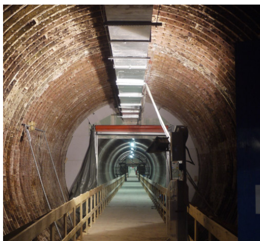
Bauarbeiten in der Oströhre des Alten Elbtunnels
